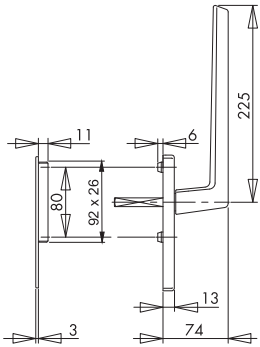
Manilla interior con uñero por la parte exterior, cuadradillo de 10mm
