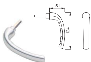
Manilla Quita Pon
