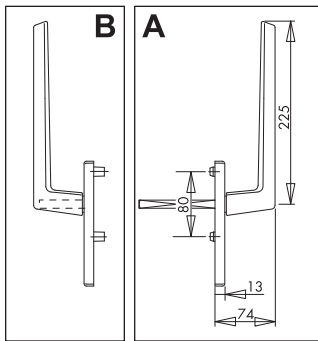
Manilla doble lado exterior con bocallave (B)
